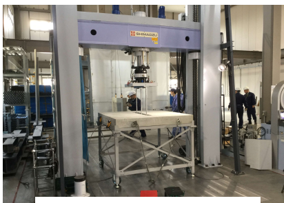
押し抜き強度(載荷試験)
